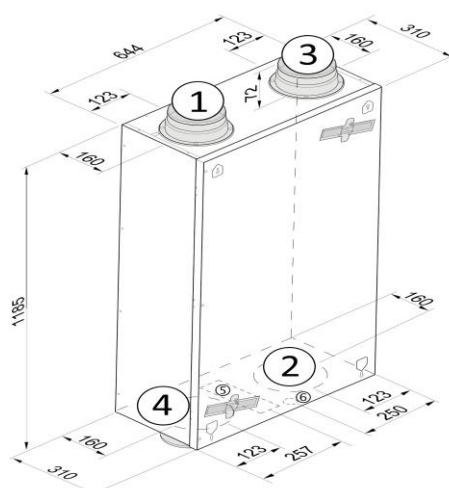
RENOVENT SKY 300
